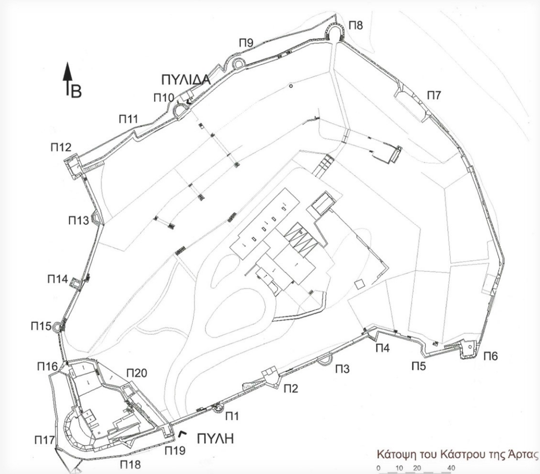
Εικ. 19. Κάτοψη του κάστρου της Άρτας – σύγχρονη αρχιτεκτονική αποτύπωση. Πηγή: Β. Παπαδοπούλου, Άρτα – Το Κάστρο, Αθήνα 2023.
