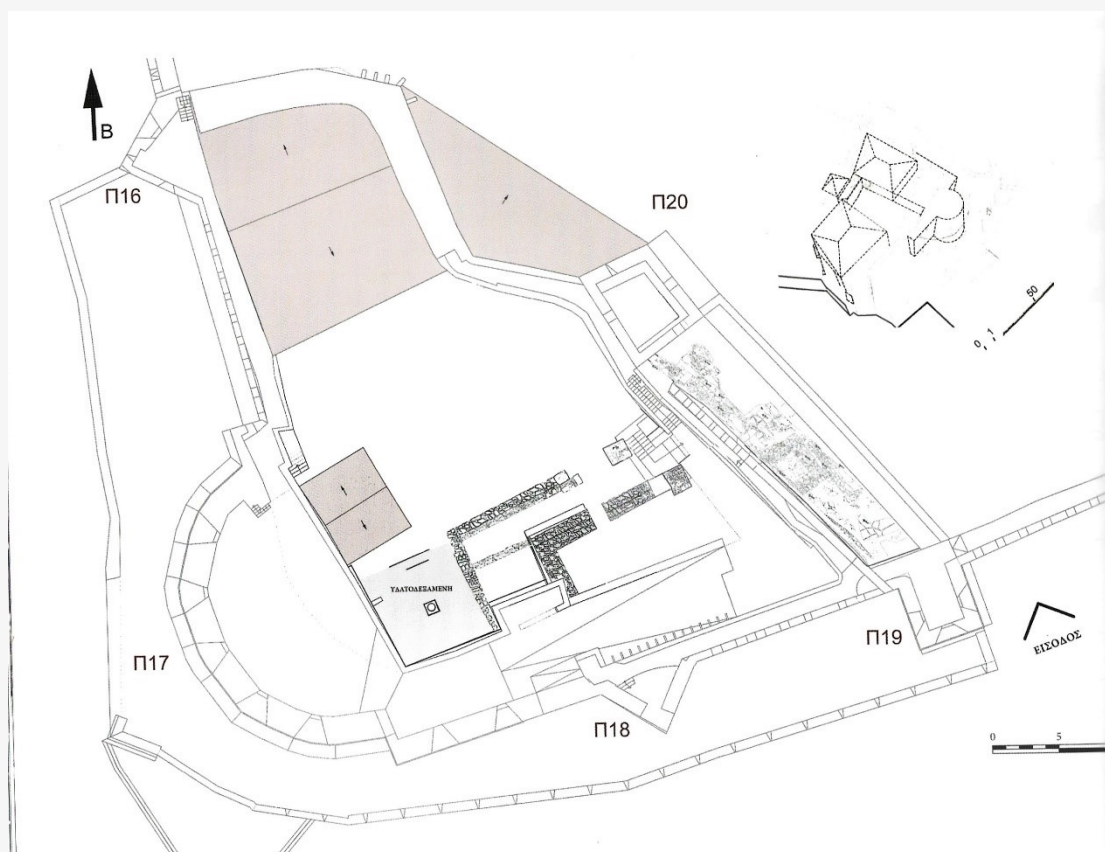
Εικ. 20. Λεπτομερής σύγχρονη αρχιτεκτονική αποτύπωση τμήματος του κάστρου της Άρτας (πύργοι Π17–Π20), με ένδειξη δομικών φάσεων και αρχαιολογικών καταλοίπων. Πηγή: Β. Παπαδοπούλου, Άρτα – Το Κάστρο, Αθήνα 2023.
